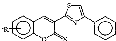
Спектрально-люминесцентные характеристики 3-(4-фенилтиазолил-2)-кумаринов и их 2-иминоаналогов в пропанол-2
